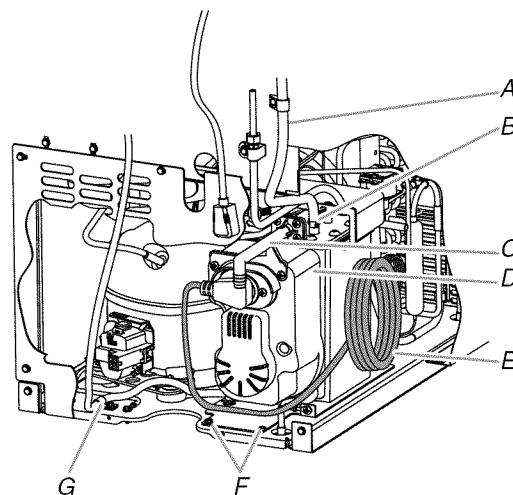
A. Tube de ventilation B. Bride de tuyau de \frac{5}{8} " C. Tuyau d'évacuation de la pompe D. Pompe de vidange E. Cordon d'alimentation de la machine à glaçons F. Vis de montage de la pompe n° 8-32 x \frac{3}{8} " G. Cordon d'alimentation de la pompe de vidange, bride et vis
