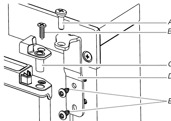
A. Axe de la charnière B. Vis Phillips fraisée C. Butée de porte
