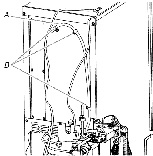
A. Tube de ventilation
