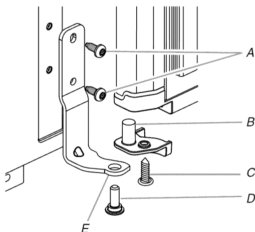
A. Vis de charnière à tête hexagonale B. Butée de porte C. Vis Phillips fraisée D. Axe de charnière E. Charnière
