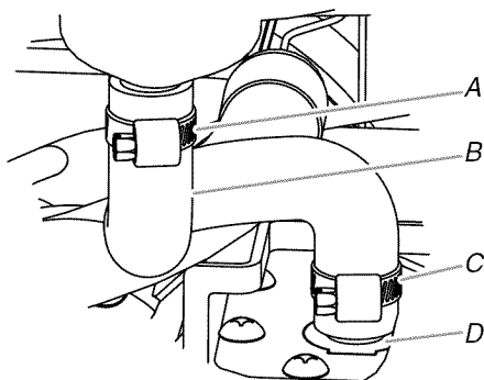
A. Bride de tuyau réglable de \frac{7}{8} " B. Tube de vidange (entre le bac à glaçons et la pompe de vidange) C. Bride de tuyau réglable de \frac{7}{8} " D. Entrée du réservoir de la pompe de vidange
